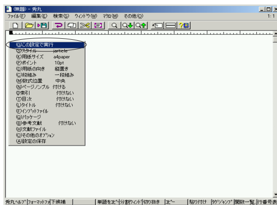
Fig. 4.4 sset2e.mac の起動
