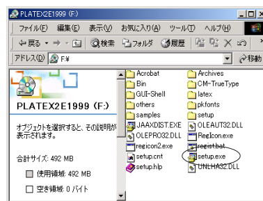
Fig. 2.1 Platex2e1999の中身
