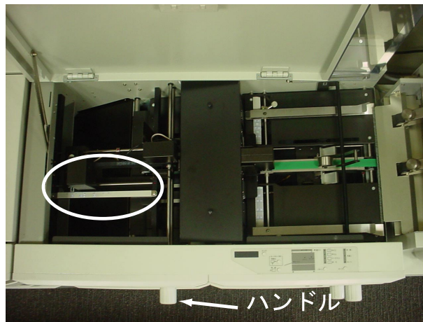
Fig. 38 中とじストッパー位置調整
