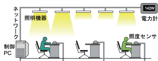
Fig.1 知的照明システムの構成図
