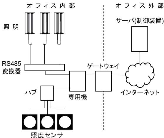
Fig.1 クラウド型知的照明システムのハードウェア構成
