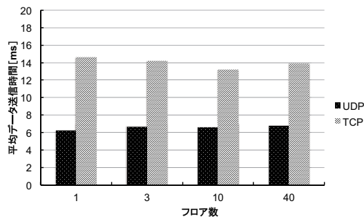
Fig.2 TCP/IP, および UDP/IP を用いた際のデータ送信平均時間の比較
