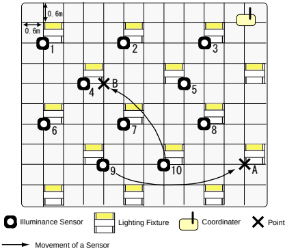
Fig.3 実験環境 (平面図)
