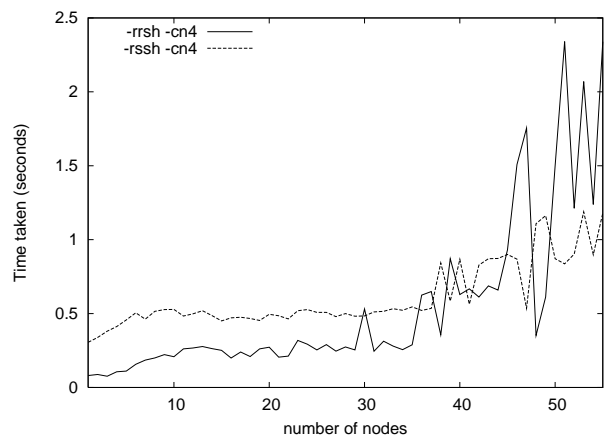
Fig. 10 階層的に実行した場合の実行結果
