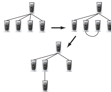
Fig. 2 downlink が多すぎる場合の再接続
