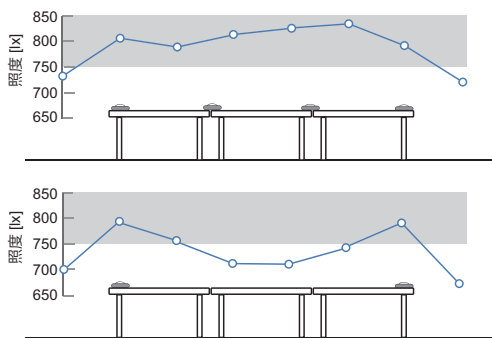
図 1: ANA/RC を用いた目標照度実現時の照度分布図
