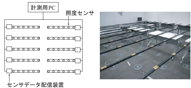
(a) 照度分布計測システムの構成 (b) 照度分布計測の様子
