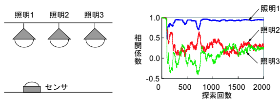
図 2: 照明と照度センサの相関
