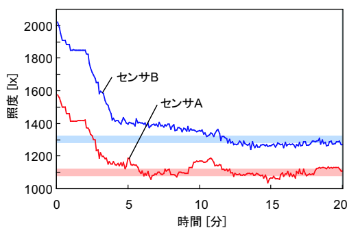
図 6: 照度履歴
