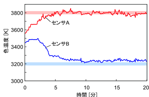
図 7: 色温度履歴
